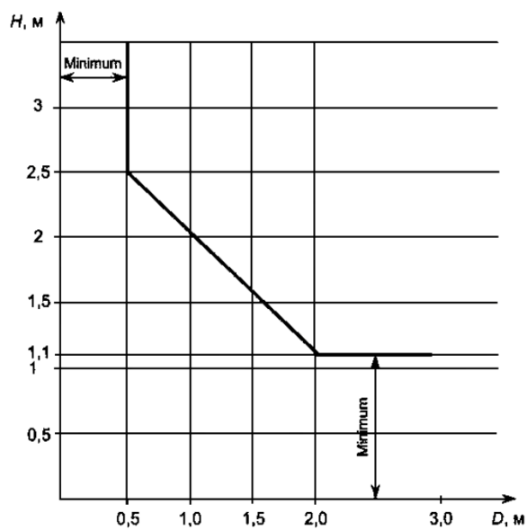
Малюнок 2 — Частково закрыта шахта. Відстані
